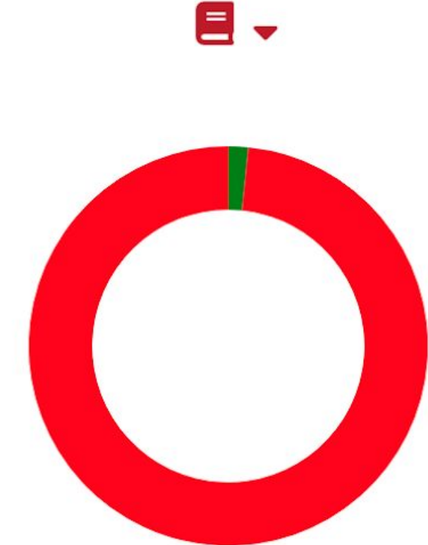
Tweet Sentiment
