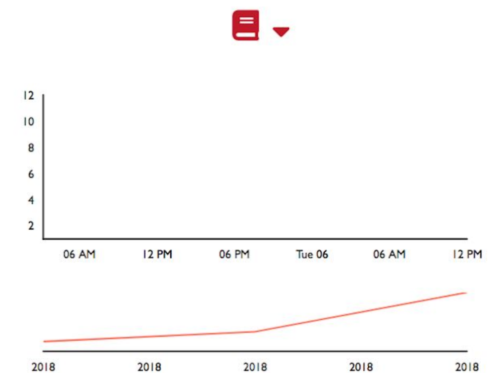
Tweet stream
